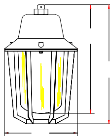
PENDANT MOUNT
